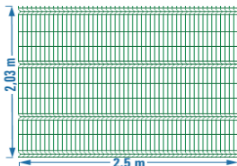
Figura 1 - Dimensões do painel do gradil
